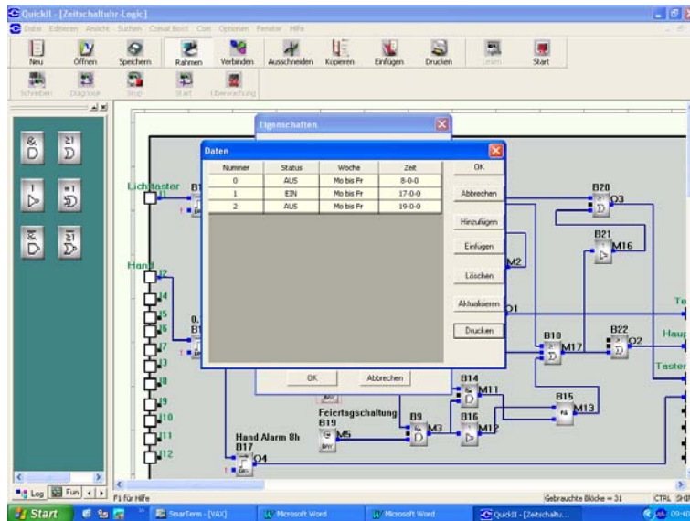
Beispiel für die Programmierung der Unterdrückung der Dauerlichteinschaltung an verkehrsarmen Tagen, Feiertagen.
